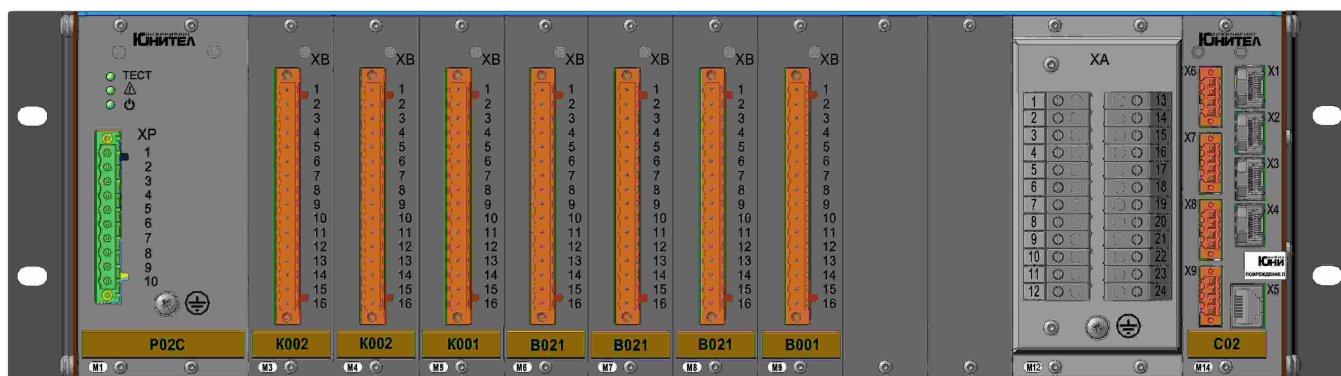
Рисунок 1.1 – Вид устройства «ЮНИТ-М319-ДЗТ2» с размещением модулей по слотам (исполнение для I архитектуры)
